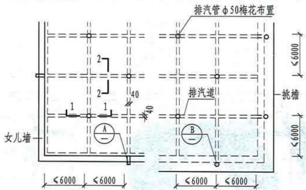
排汽道、排汽管平面布置图
