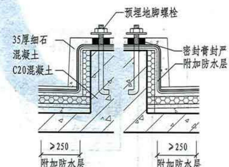
④ 设备基座
