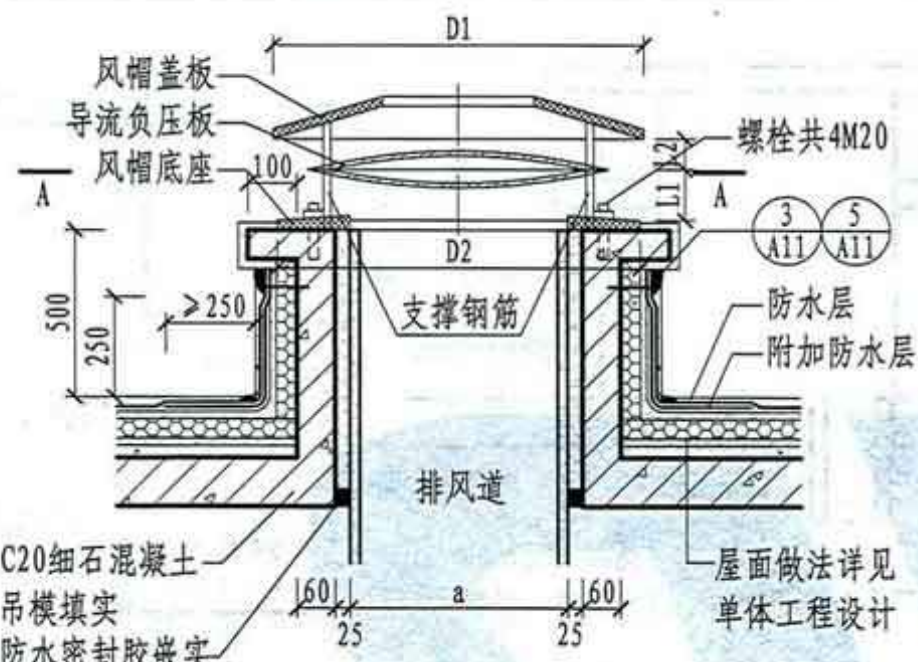
变压式风帽出屋面做法
