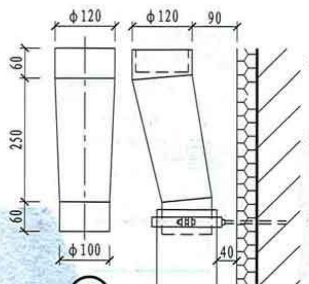
③ 圆雨水接口
