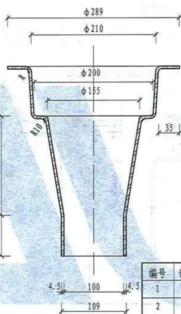
② 短管剖面图
