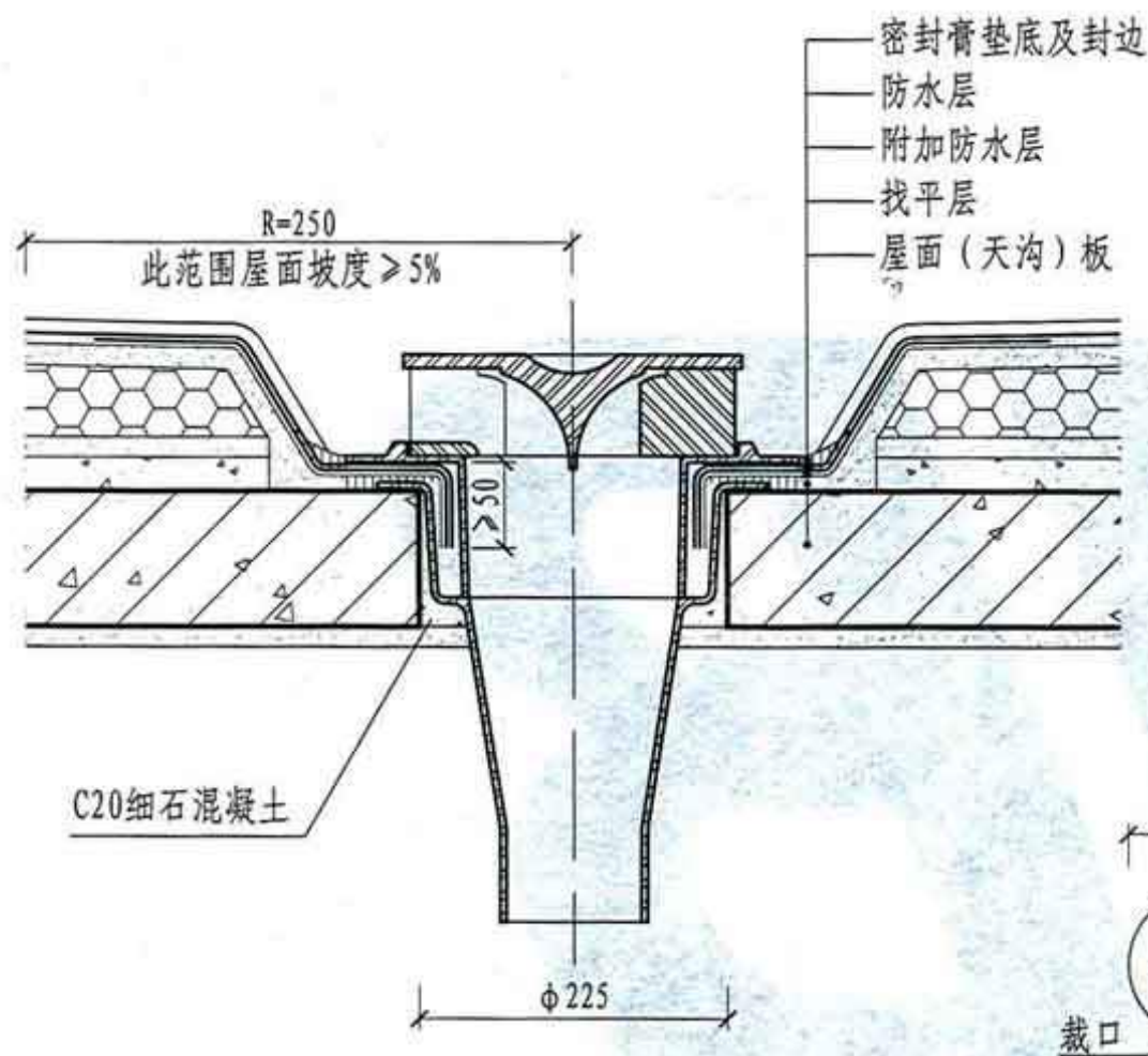
① 屋面(天沟)板上安装(一)
