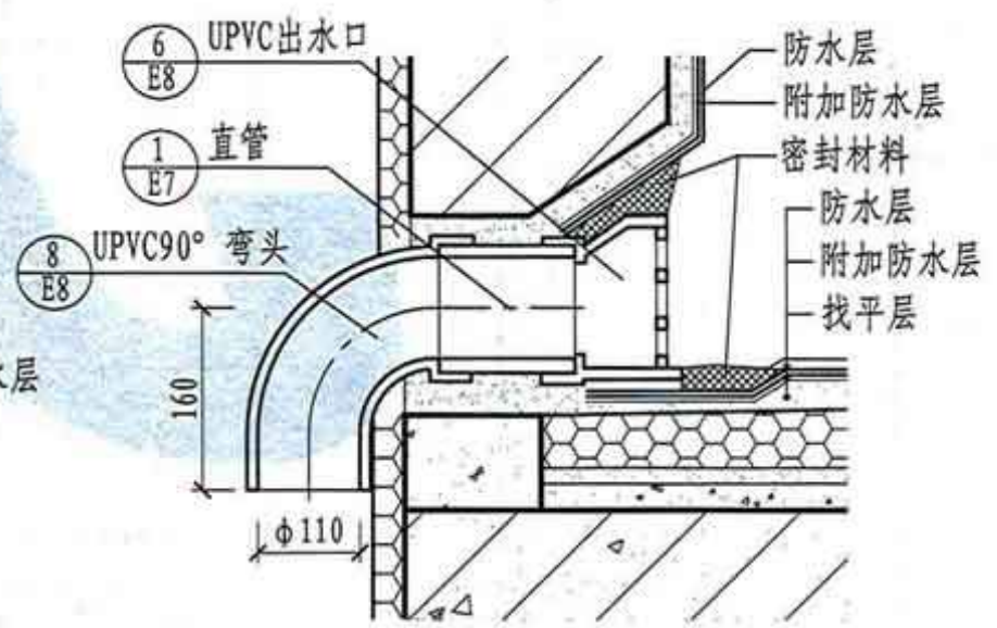
⑥ 女儿墙UPVC雨水口
