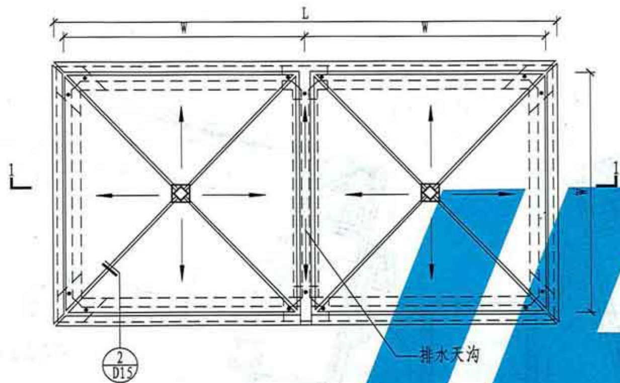
隐框四面锥采光顶平面示意图
