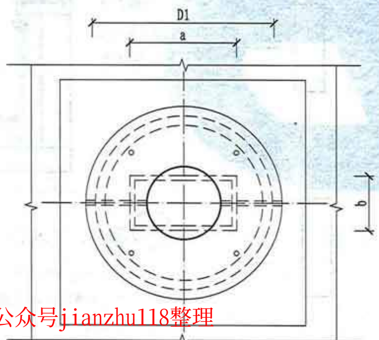
A-A变压式风帽平面图
