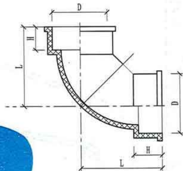
⑧ UPVC90° 弯头
