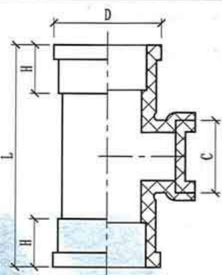
② UPVC检查口
