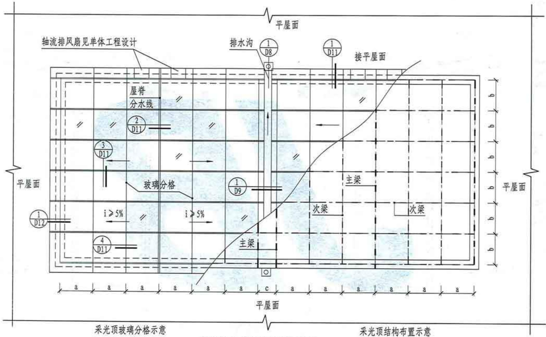
半隐框玻璃采光顶详图索引
