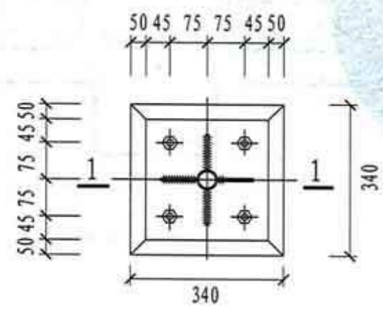
④ 屋面旗杆座俯视图
