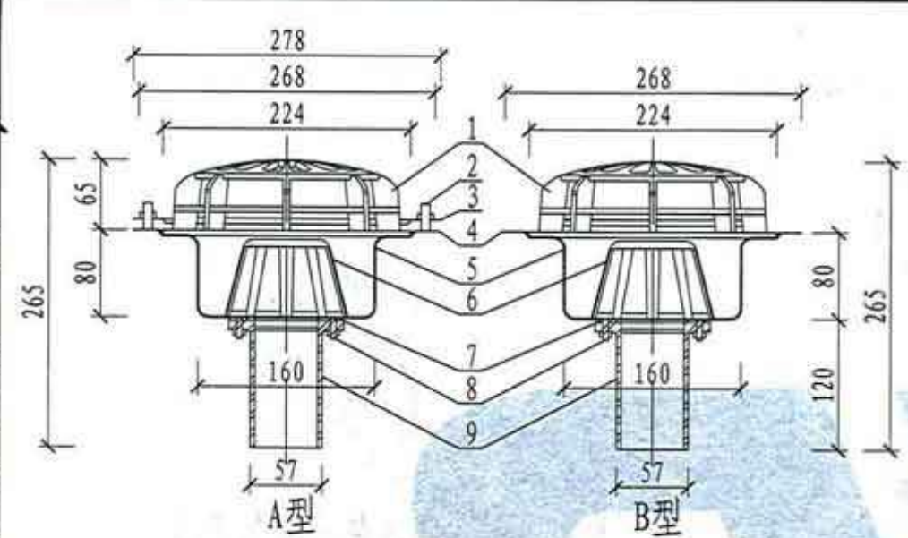
① YG50型虹吸式雨水斗
