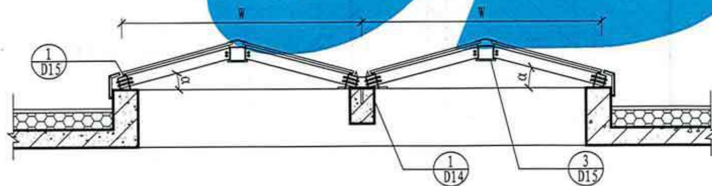
1-1剖面图
