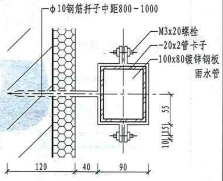
⑥ 方雨水管及卡子
