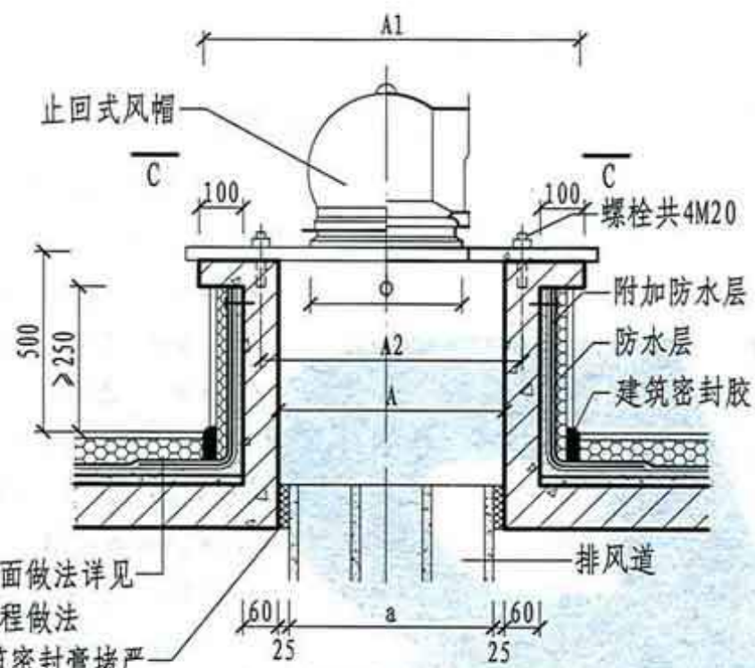
止回式风帽出屋面做法
