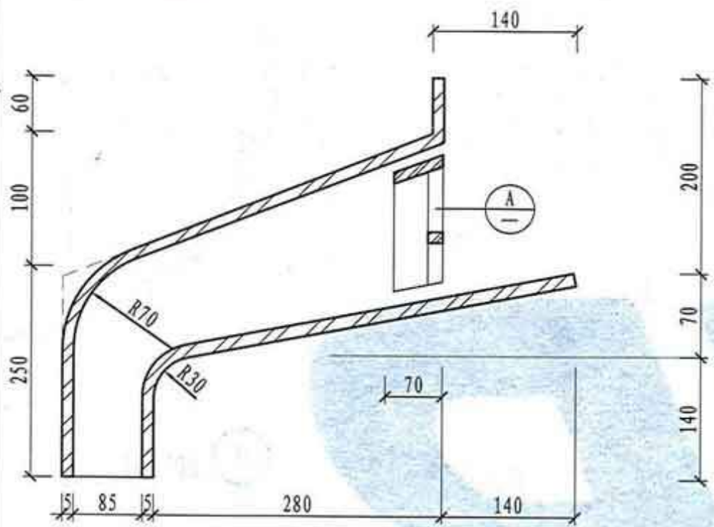
1-1剖面
