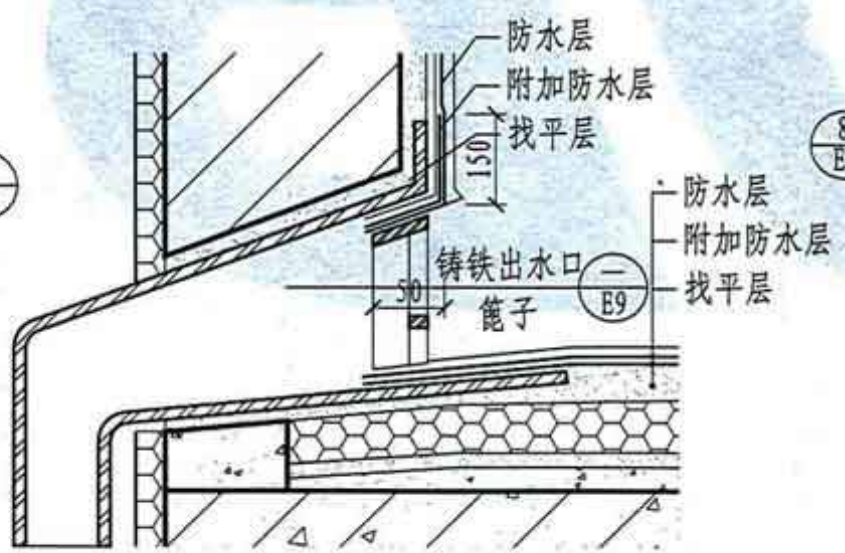
⑤ 女儿墙铸铁雨水口
