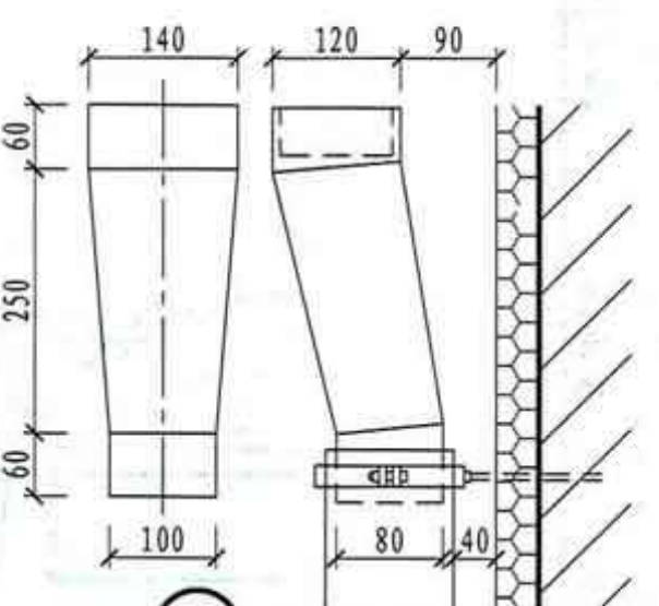
④ 方雨水接口
