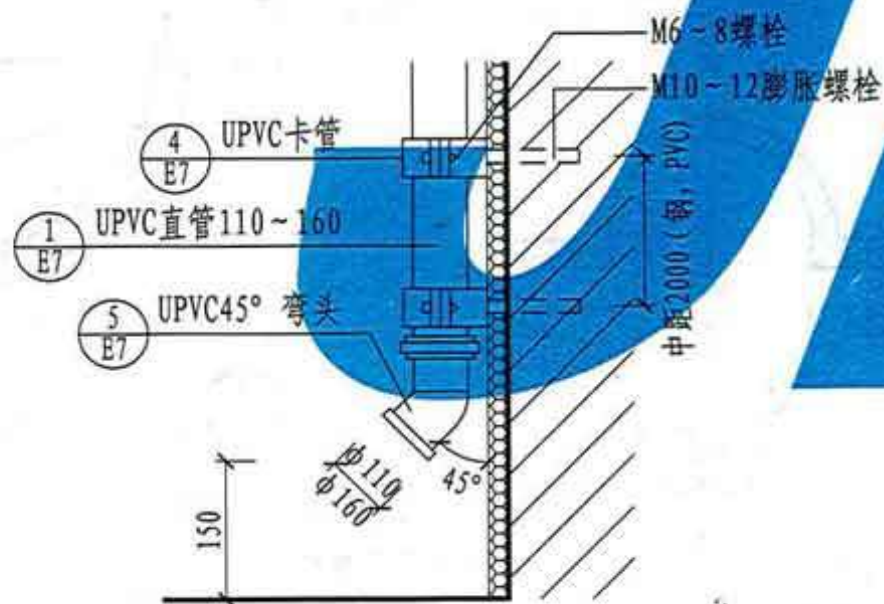
② 外排UPVC管底出水口
