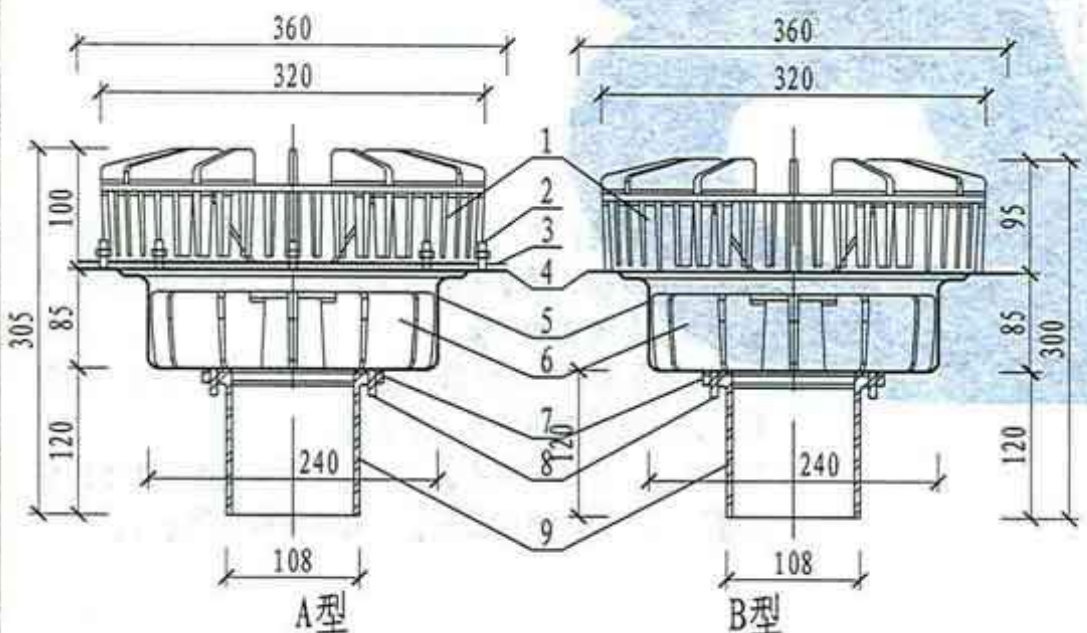
③ YG100型虹吸式雨水斗
