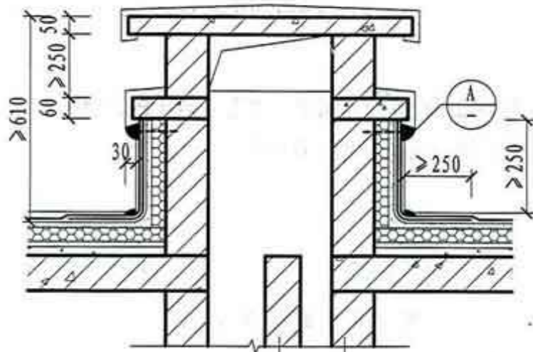
1-1 当用砌块砌风道、烟囱时，通风道外壁顶住楼板
