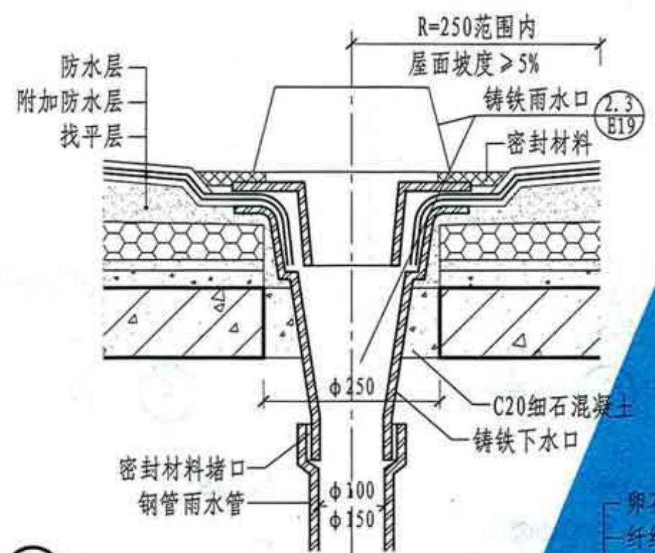
⑤ 内排水铸铁雨水口
