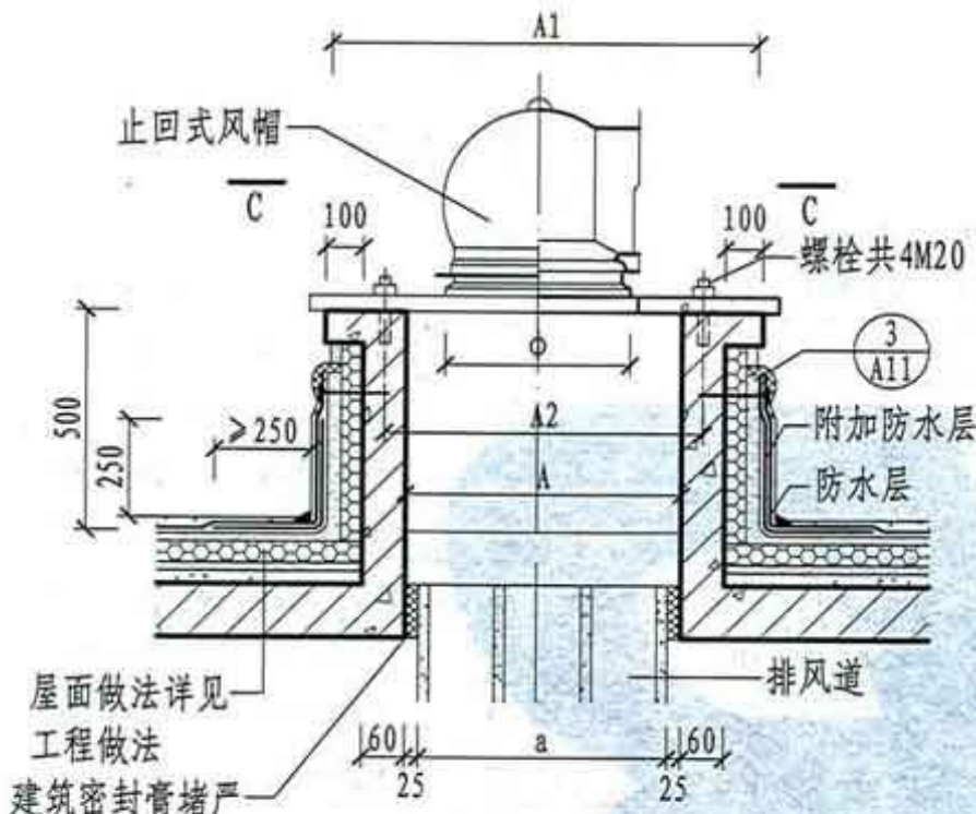
止回式风帽出屋面做法
