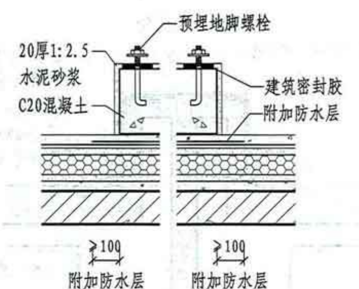
③ 轻型设备基座
