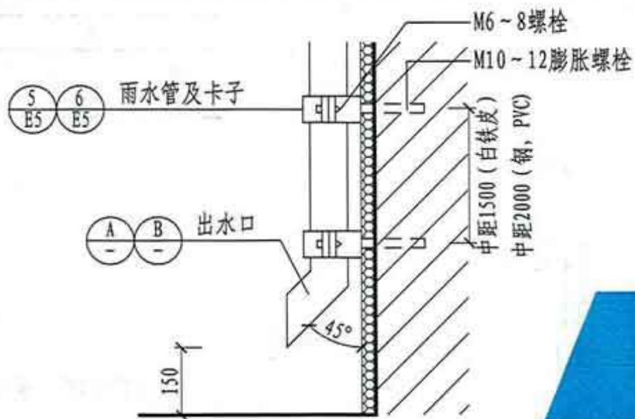
① 外排镀锌钢板管底出水口
