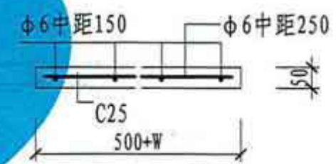
GB-1配筋图
