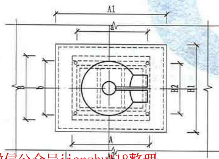
C-C止回式风帽平面图
