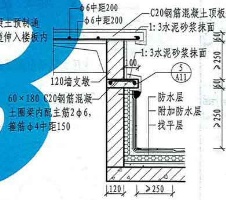
A 烟囱、通风道出屋面节点
