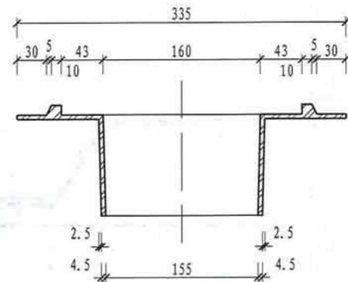
③ 环形筒剖面图
