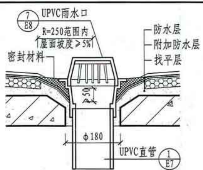
③ 挑檐UPVC雨水口
