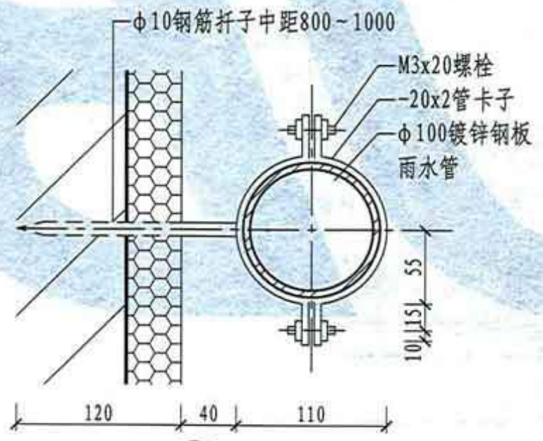
⑤ 圆雨水管及卡子
