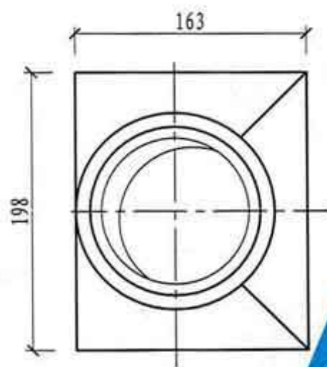
⑥ UPVC外雨水口
