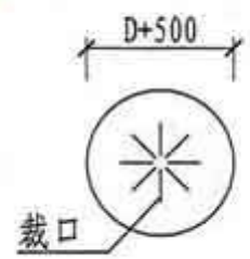
雨水口附加防水层叉面裁剪图
