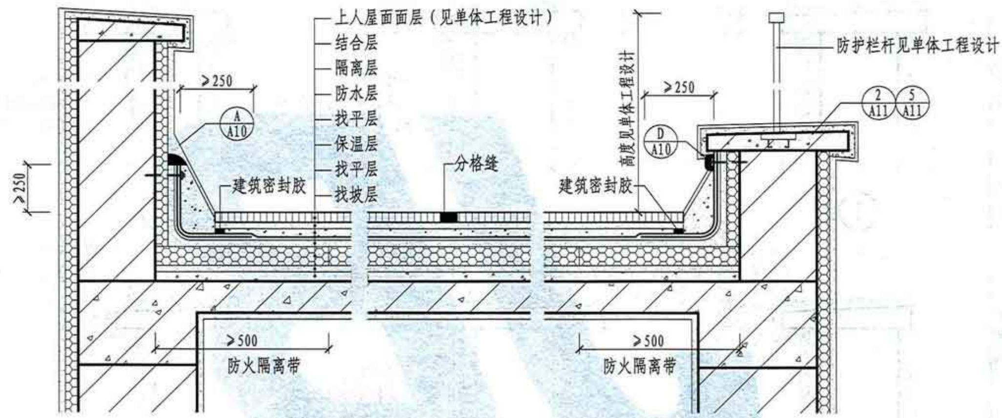
① 女儿墙处屋面泛水
