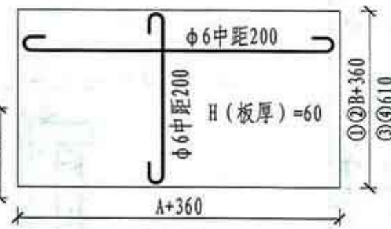
顶板构造
