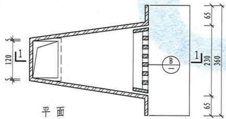
外雨水口篦子
