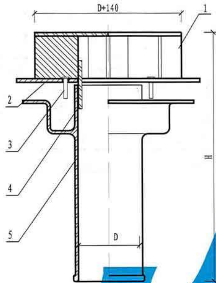
① 铸铁短管雨水斗总装配图
