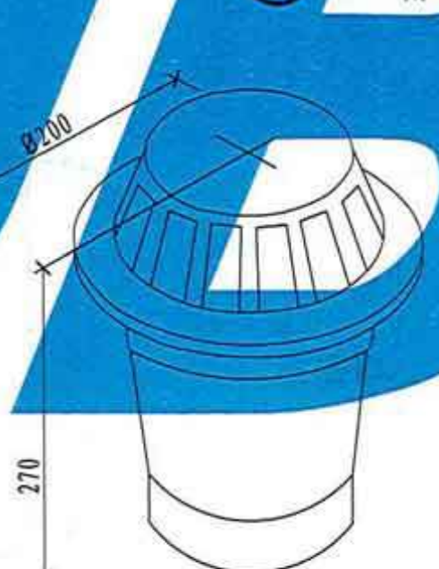
⑦ UPVC雨水口
