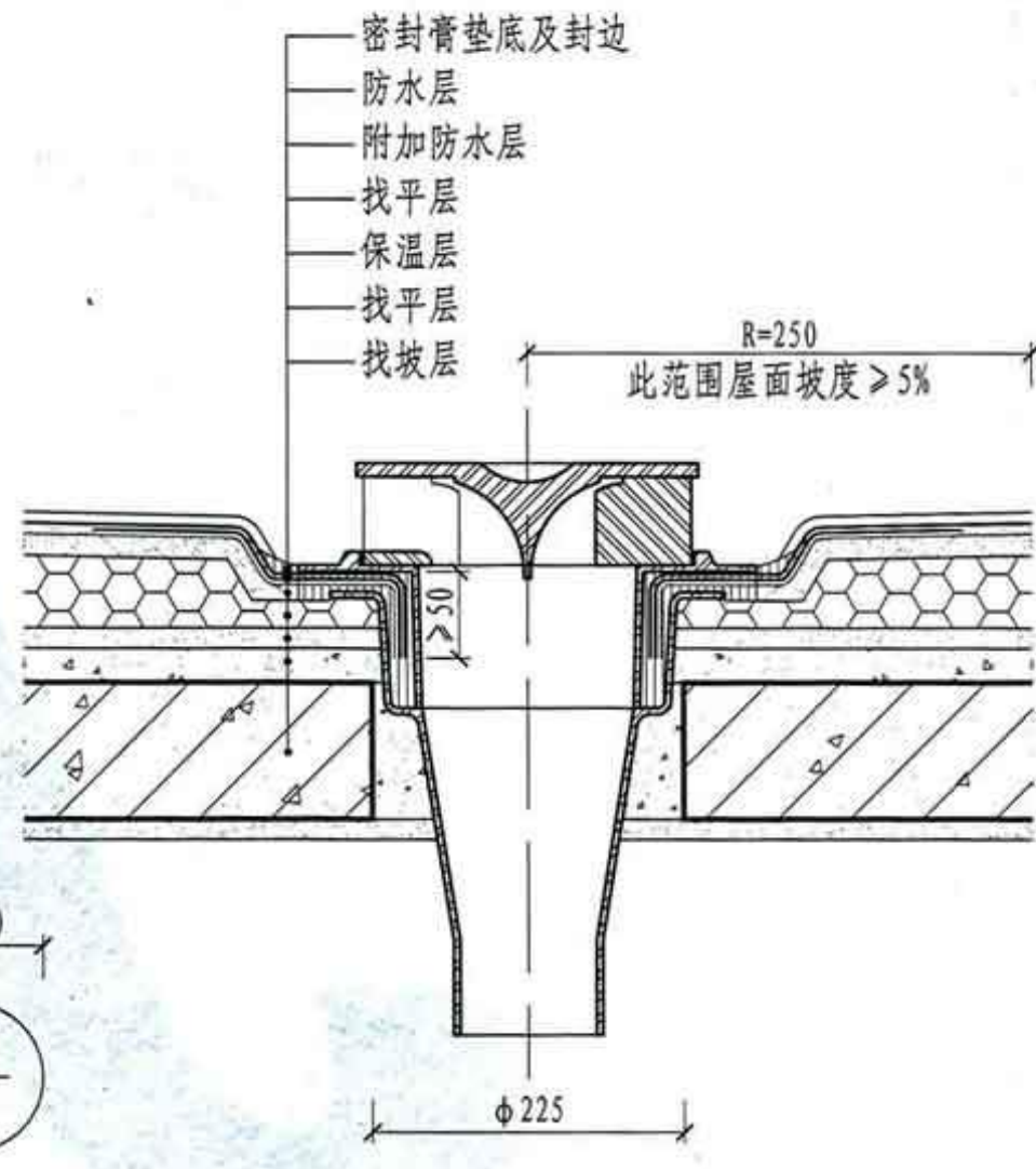
② 屋面(天沟)板上安装(二)
